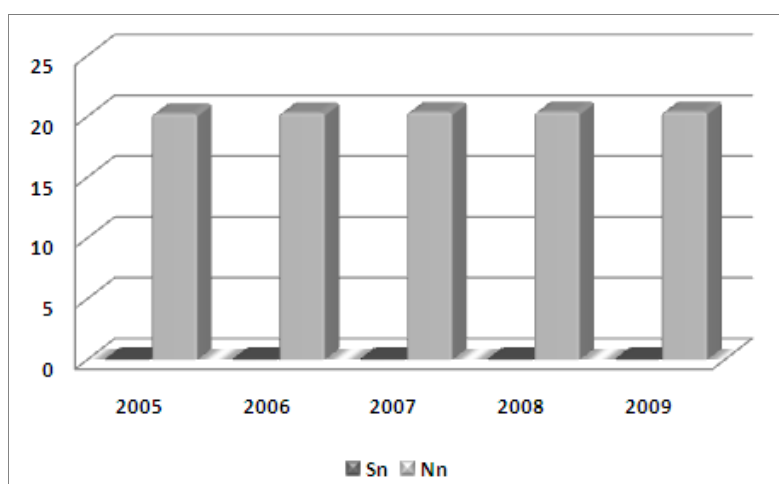
Rysunek 7. Zapotrzebowanie na moc na terenie gminy Jednoróżec w latach 2005-2009 [MW].
