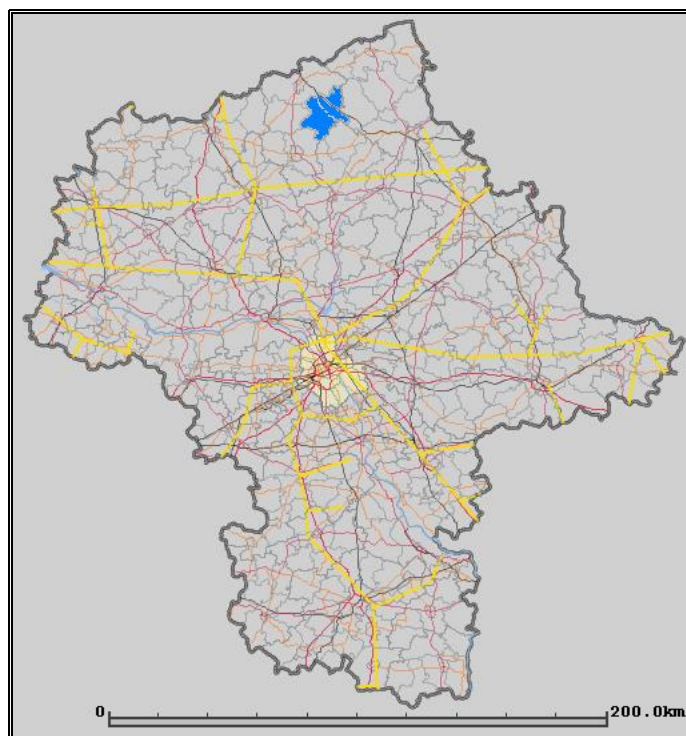
Rysunek 5. Gazociąg na terenie województwa mazowieckiego
